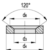
DIN 6319-D (d4=d2)
